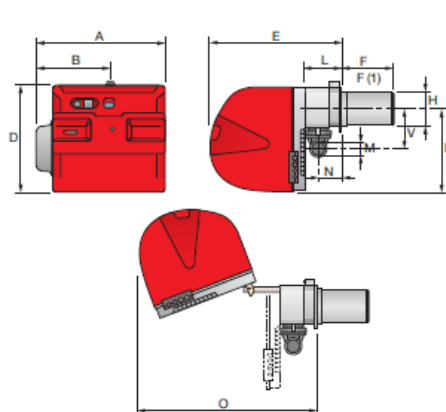
RS 64/M MZ
