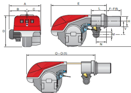
RS 70/M - 100/M - 130/M - 190/M - 250/M MZ
