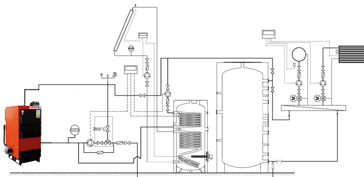
Schema de Principiu 4. Legarea cazanului SONTEC cu boiler cu 2 Serpentine, buffer, panou – colector solar și ventil cu trei căi.
