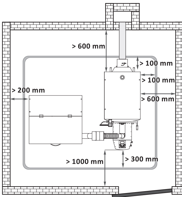
Schemă 1. Distanță recomandată a cazanului de pește față de pereți
