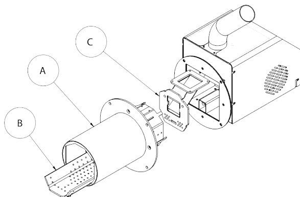
Schemă 8. Se demonteaza corpusul camerei de ardere
