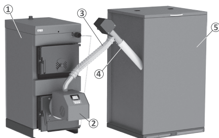
Schemă 5. Cazanul pe peleți WBC cu arzător Pell ECO
